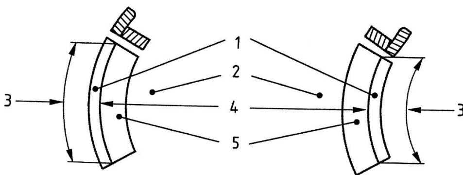
a) krawężnik łukowy „wkłęsły”
