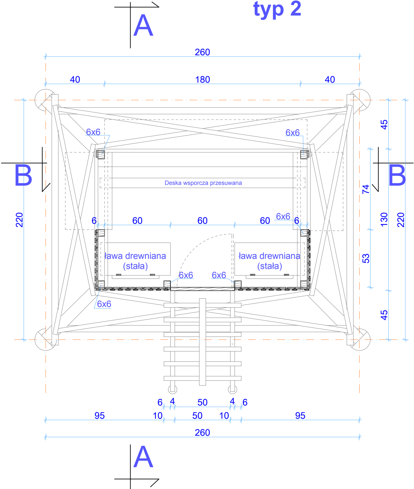
RZUT POZIOMY SKALA 1:20
