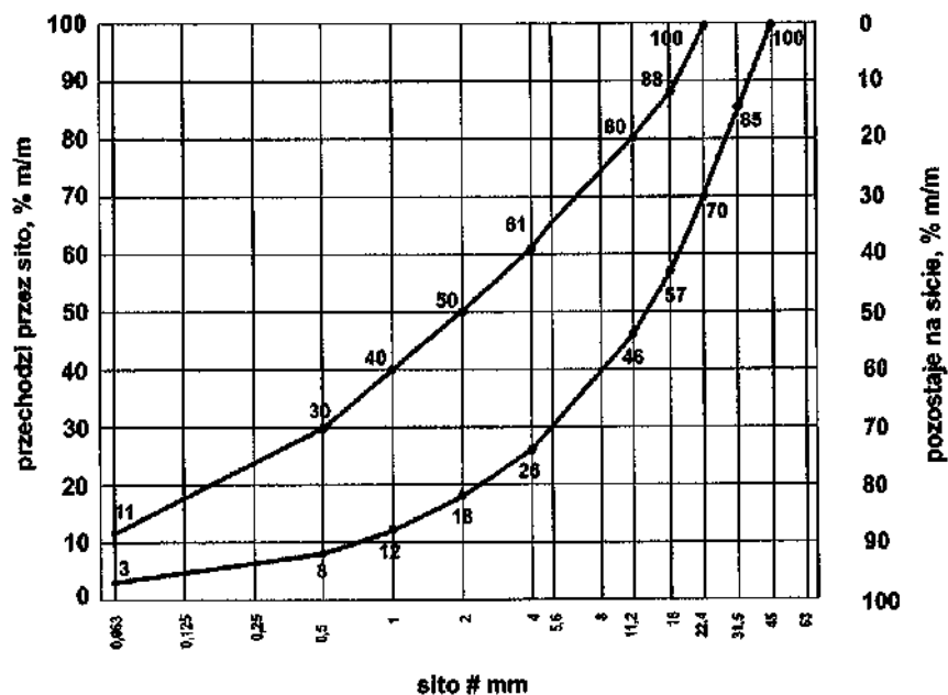
Rys. 1. Krzywe graniczne uziarnienia mieszanki mineralnej 0/31,5 m
