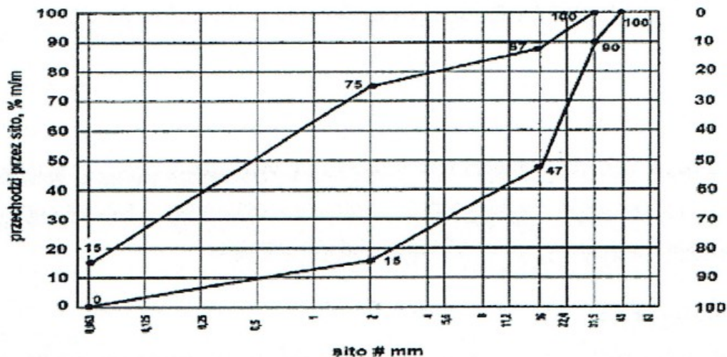
Rys. 1. Mieszanka niezwiązana 0/31,5 do nawierzchni z kruszywa niezwiązanego
