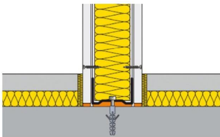
Prawidłowe połączenie ściany działowej ze stropem.
