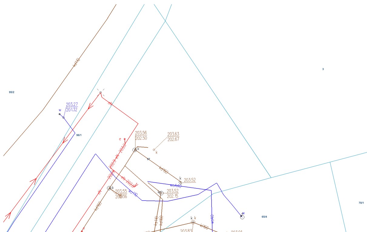
Rysunek 2 Lokalizacja sieci wodociągowej, kanalizacyjnej i energetycznej
