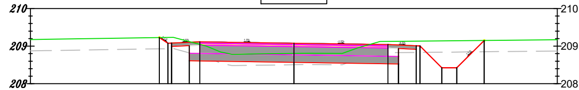
dr 347018T 0+550.000
