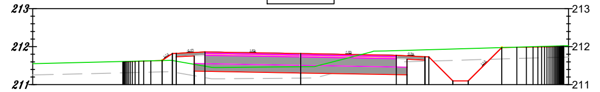
dr 347018T 0+475.000
