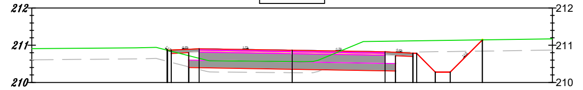
dr 347018T 0+500.000
