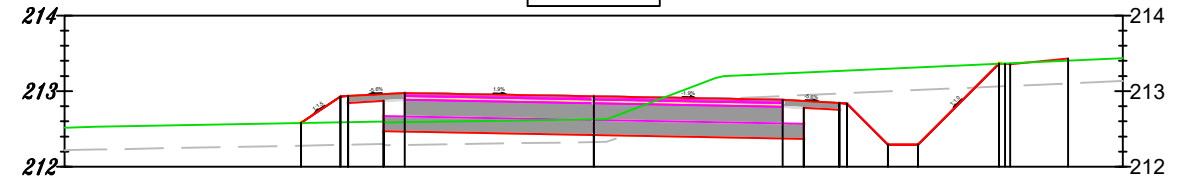
dr 347018T 0+450.000
