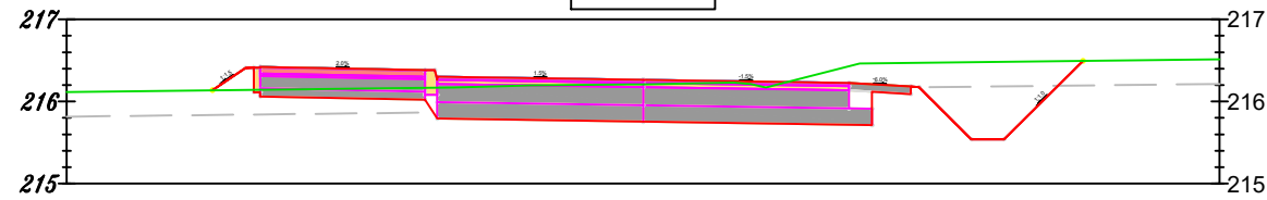
dr 347018T 0+350.000
