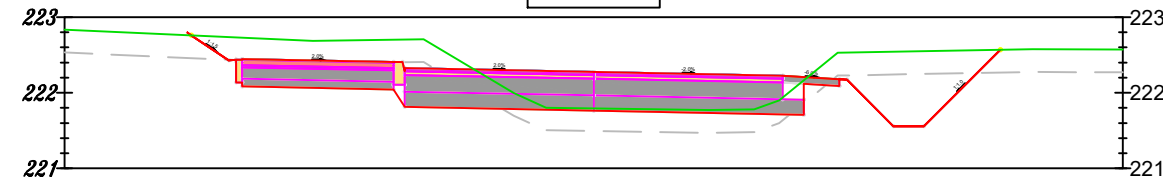
dr 347018T 0+250.000
