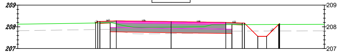
dr 347018T 0+575.000
