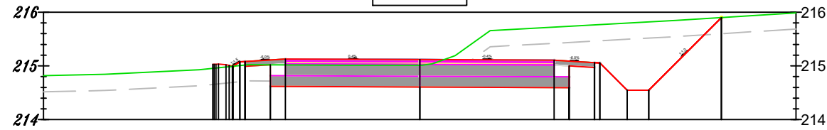
dr 347018T 0+400.000
