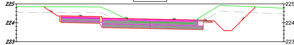
dr 347018T 0+225.000
